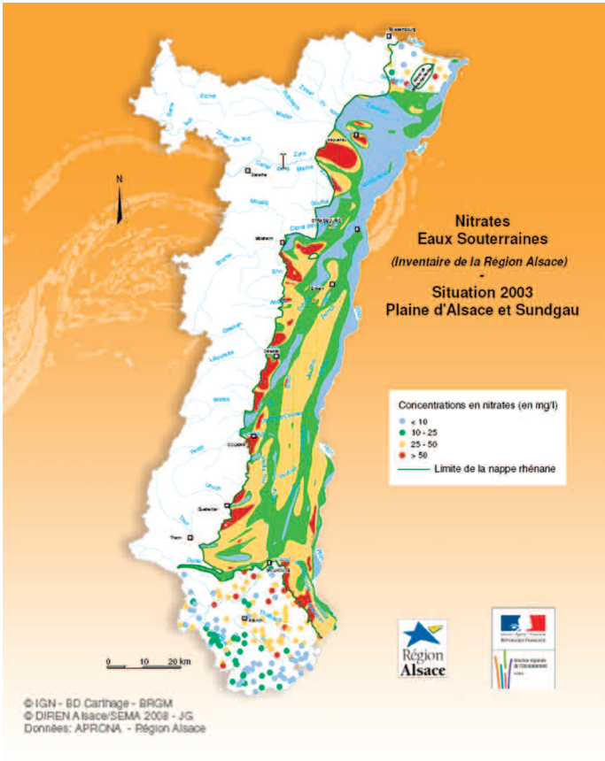
Concentrations en nitrates dans la nappe d'Alsace – situation en 2003.
